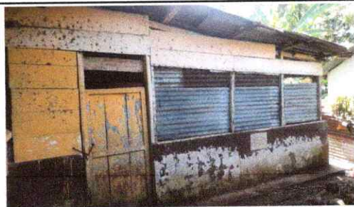
FOTO 5: Sustrucción de lámina, por lámina troquelada aluzinc calibre 26 y estructura portante (MODULO AULA II)
